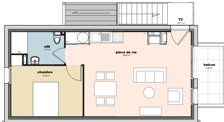
PLAN DU LOGEMENT NIVEAU 1
