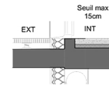
Coupe de principe accès balcon
